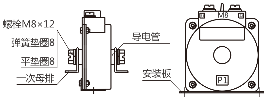
图5 安装板固定： M8和Φ8型、Φ12型
